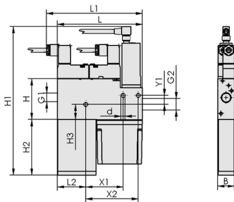
Données de construction SCP 25 NC AS RD
