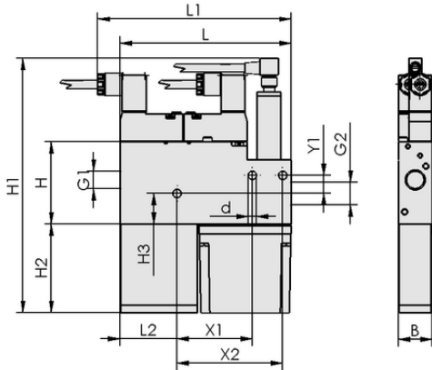
Tasarım verileri SMP 20 NC AS RD
