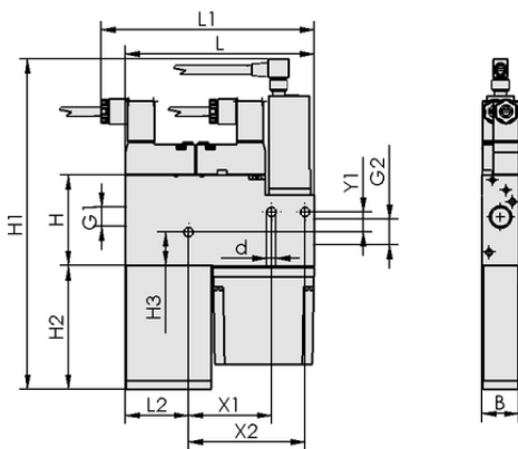
Données de construction SCP 30 NC AS VD
