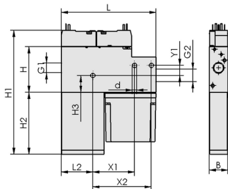
Données de construction SCP 25 NO AS
