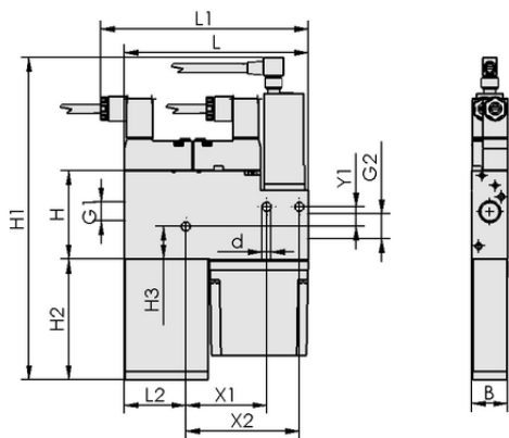
Données de construction SCP 20 NO AS VD
