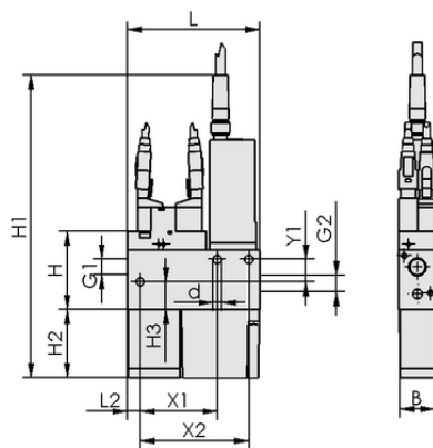
Données de construction SCP 10 NO AS VD
