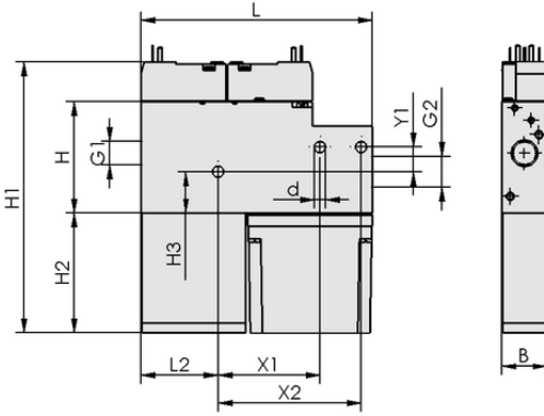
Tasarım verileri SMP 30 NO AS
