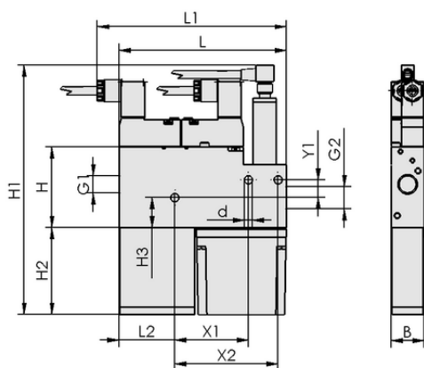
Dati di costruzione SMP 25 NO AS RD
