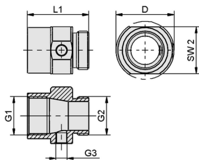
Dati di costruzione VRL-R NPT1 50.3x39 AL
