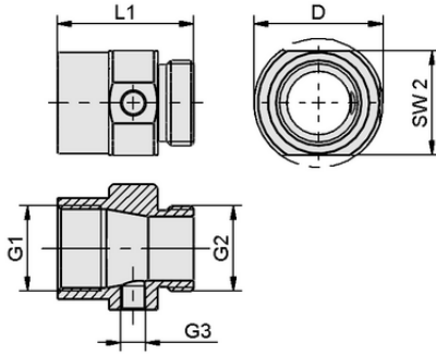
Tasarım verileri VRL-R G3/4 44.5x39 AL
