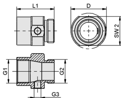
Dati di costruzione VRL-R G3/4 44.5x39 AL
