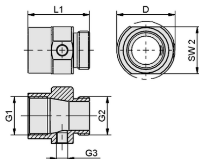
Données de construction VRL-R G3/4 44.5x39 AL
