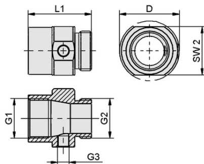
Données de construction VRL-R NPT3/4 44.5x39 AL
