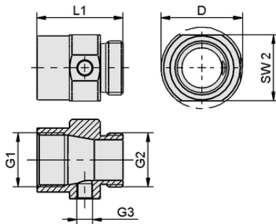
デザインデータ VRL-R NPT3/4 44.5x39 AL
