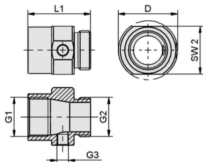
Dati di costruzione VRL-R NPT3/4 44.5x39 AL
