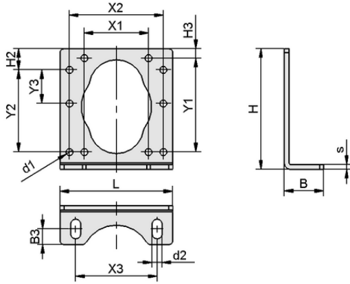
Tasarım verileri BEF-WIN 72x25x77 SBPL/SCPL
