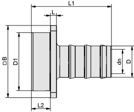
Tasarım verileri ST 32 AL-EL
