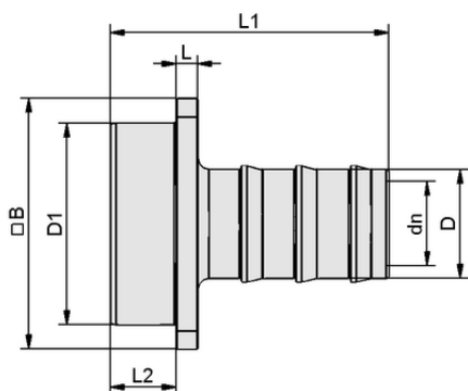
Dati di costruzione ST 32 AL-EL
