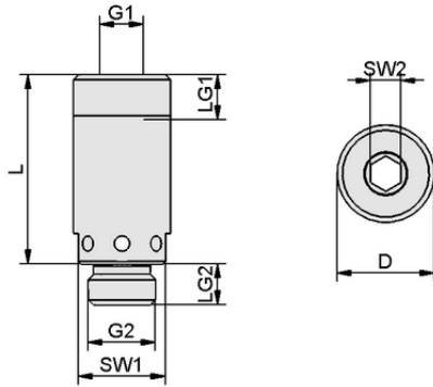
Tasarım verileri SEV G1/8-IG G1/8-AG
