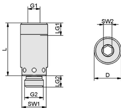
デザインデータ SEV G1/8-IG G1/8-AG
