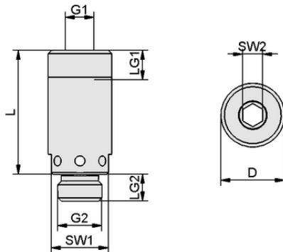
デザインデータ SEV G1/8-IG G1/4-AG
