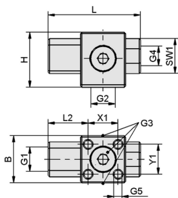
Données de construction SFE 7 AL
