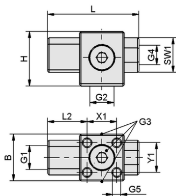
デザインデータ SFE 7 AL
