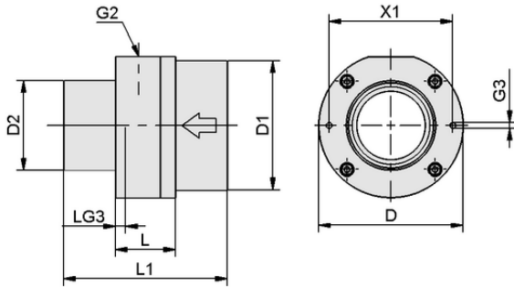
Tasarım verileri SEC-60 A2
