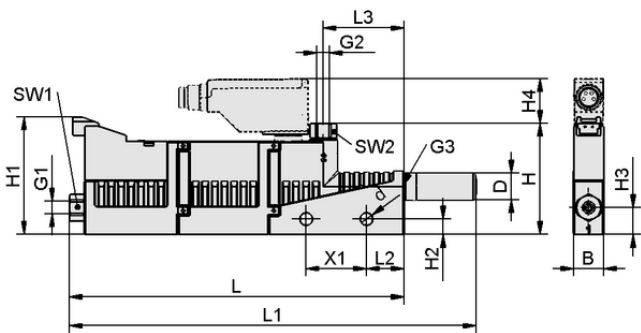
Design data SBP-C 07 G01 NC AI VS-T
