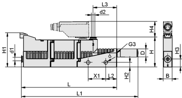
Design data SBP-C 07 S01 NC AI VS-T
