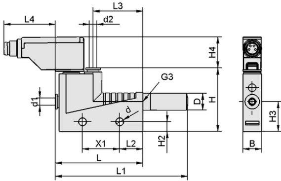
Tasarım verileri SBP-C 25 S03 VS-T
