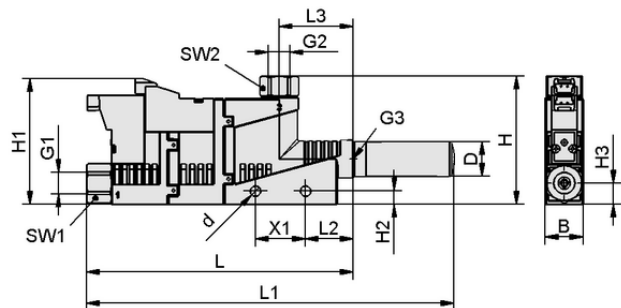
Données de construction SBP-C 07 G01 NC
