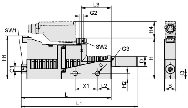
Données de construction SBP-C 05 G01 NC
