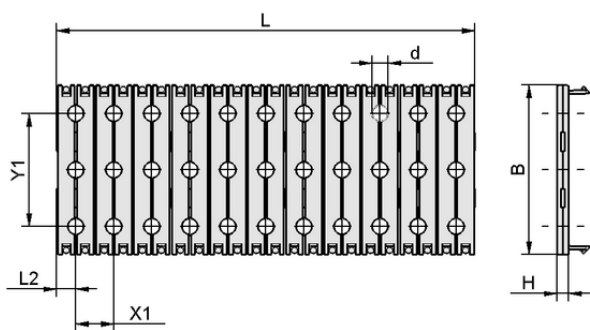
デザインデータ BEF-PL 110x44.5x3 SBP
