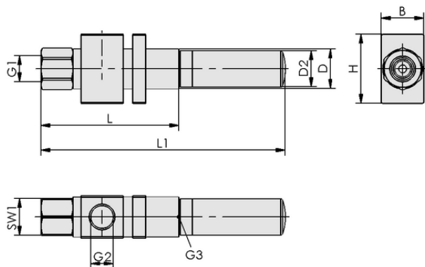
Dati di costruzione SEG 07 HS-S SDA
