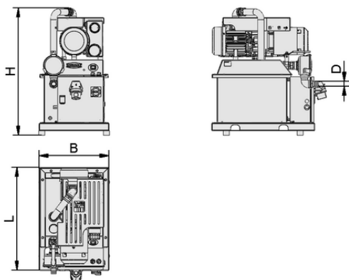
Données de construction VH-OG Plus 100 100
