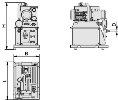
Dati di costruzione VH-OG Start 100 100
