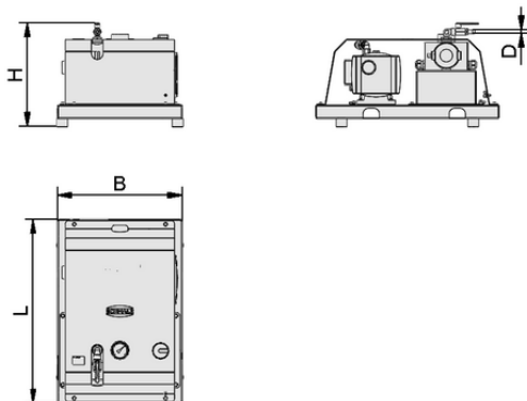
Dati di costruzione VH-OG Start 10 10
