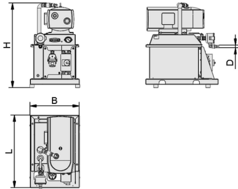
Tasarım verileri VH-TR Start 25 30
