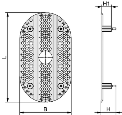
Tasarım verileri LOCH-PL 235x135x39 ST PSSG
