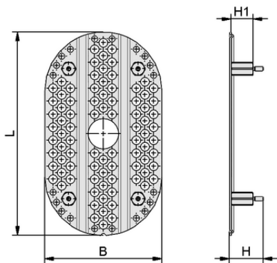
デザインデータ LOCH-PL 235x135x29 ST PSSG
