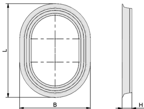
Données de construction DR-PSSG 350x250 NBR-60
