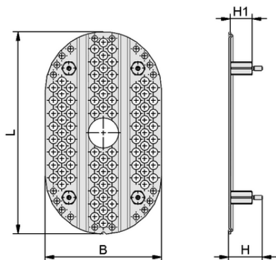
デザインデータ LOCH-PL 288x188x31.5 ST PSSG
