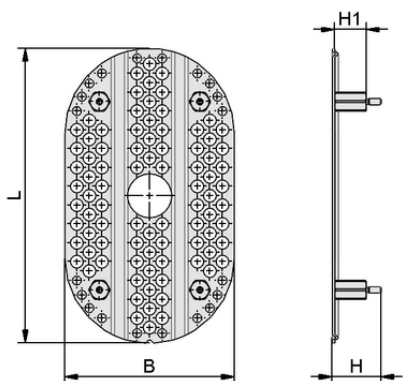
Dati di costruzione LOCH-PL 288x188x44 ST PSSG
