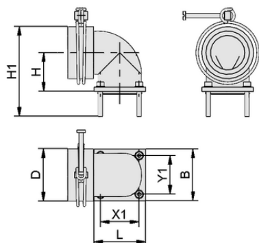
デザインデータ SCHL-AN W 32.5-47x47x35 PSSG
