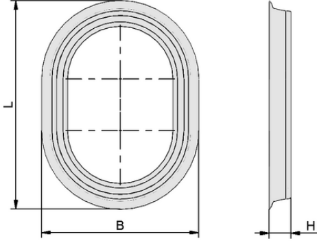
Tasarım verileri DR-PSSG 290x215 NBR-60
