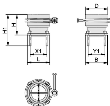
デザインデータ SCHL-AN 32.5-47x47x48 PSSG
