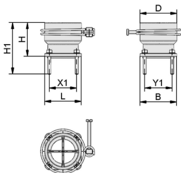
Datos de diseño SCHL-AN 32.5-47x47x48 PSSG
