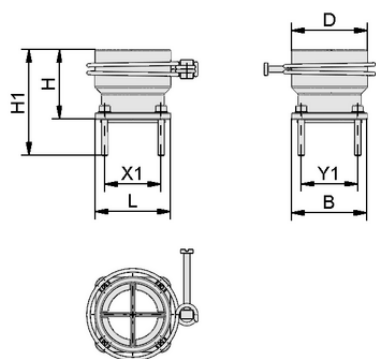
Datos de diseño SCHL-AN 60.5-60x60x55 PSSG
