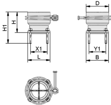
Tasarım verileri SCHL-AN 60.5-60x60x55 PSSG
