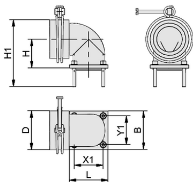
Datos de diseño SCHL-AN W 60.5-60x60x45 PSSG
