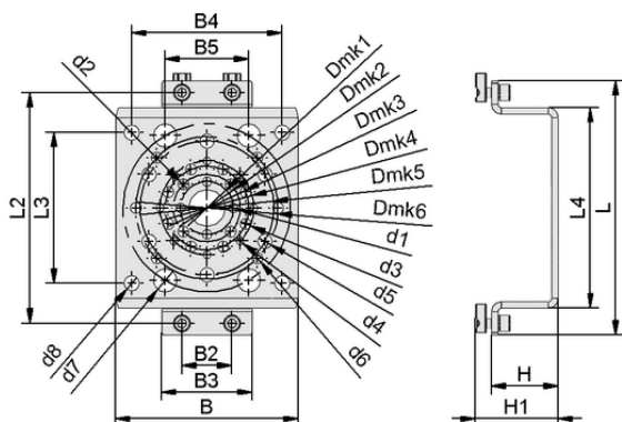
デザインデータ MOD-FLAN 152x109 FXP/FMP-60
