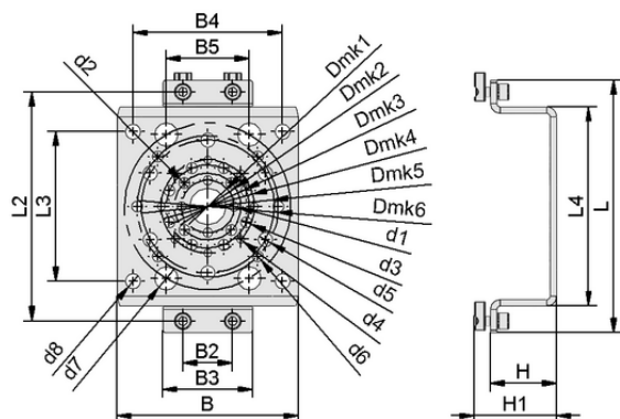
Dati di costruzione MOD-FLAN 152x109 FXP/FMP-60
