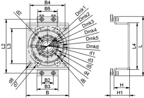
Tasarım verileri MOD-FLAN 152x109 FXP/FMP-60
